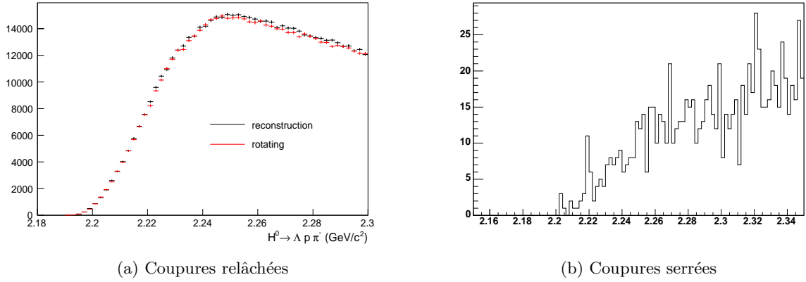
FIG. 4.20 – Spectres en masse invariante de \Lambda p \pi^- , données Au-Au à 200 \text{GeV} , déclenchement Central .
