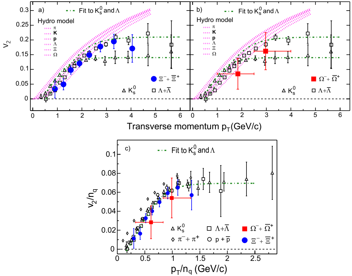
FIG. 2.16 – Flow elliptique des particules \pi , K , p , \Lambda , \Xi et \Omega en fonction de la p_T , sans et avec normalisation au nombre de quarks constituant n_q . Les prédictions de l'hydrodynamique sont représentées en pointillés roses [23].
