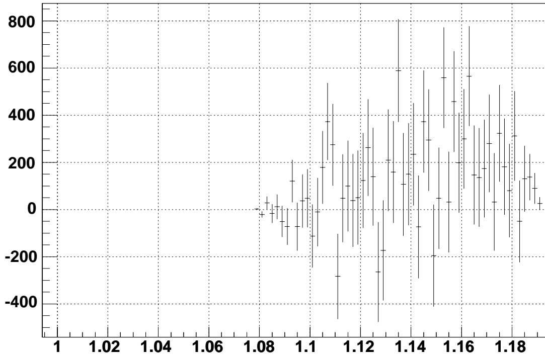
FIG. A.8 – Spectre de m_{\Lambda p \pi^-} - m_{\Lambda} pour les coupures du tableau A.6.
