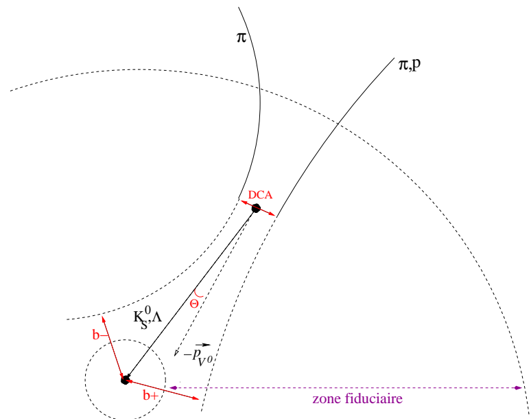
FIG. 5.2 – Topologie de désintégration en V^0 .
