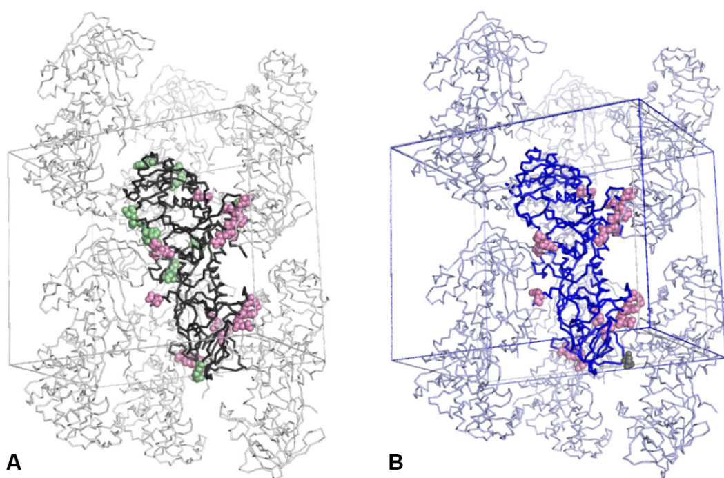
Figure II. 22 : Illustration des contacts cristallins impliqués dans l'empilement pour la GlnRS-Dr native (gris, A ) ou co-cristallisée en présence de petits substrats. (bleu, B ) Les contacts sont représentés par des sphères roses pour les contacts conservés dans les trois structures, et vertes et grises pour ceux uniquement trouvés dans la structure native ou en présence de petits substrats, respectivement.
