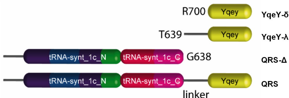
Figure II. 5 : Représentation schématique des 4 variants de la GlnRS : YqeY- \delta , YqeY- \lambda , GlnRS- \Delta et GlnRS native. Les résidus terminaux de chacun d'entre eux sont précisés. Le domaine additionnel YqeY est représenté en jaune.
