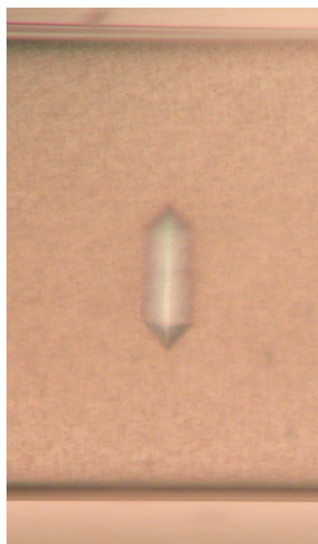
Figure III. 4 : exemple d'un cristal orienté de GlnRS-Dr. Le diamètre du capillaire est de 0,5 mm.
