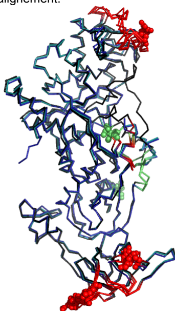
Figure II. 21 : Mise en évidence des régions comportant les variations de distances C \alpha -C \alpha pour l'enzyme Native la fGlnRS et la GlnRS/ QSI. Les distances illustrées sont celles comprises entre 2 et 3 Å, sans tenir compte de la boucle d'insertion ins2. Les régions colorées en rouge correspondent à celles présentant des distances GlnRS native-GlnRS/fGlnRS ou native-GlnRS/QSI > 2Å, celle en vert des distances entre fGlnRS et GlnRS/QSI > 2 Å.
