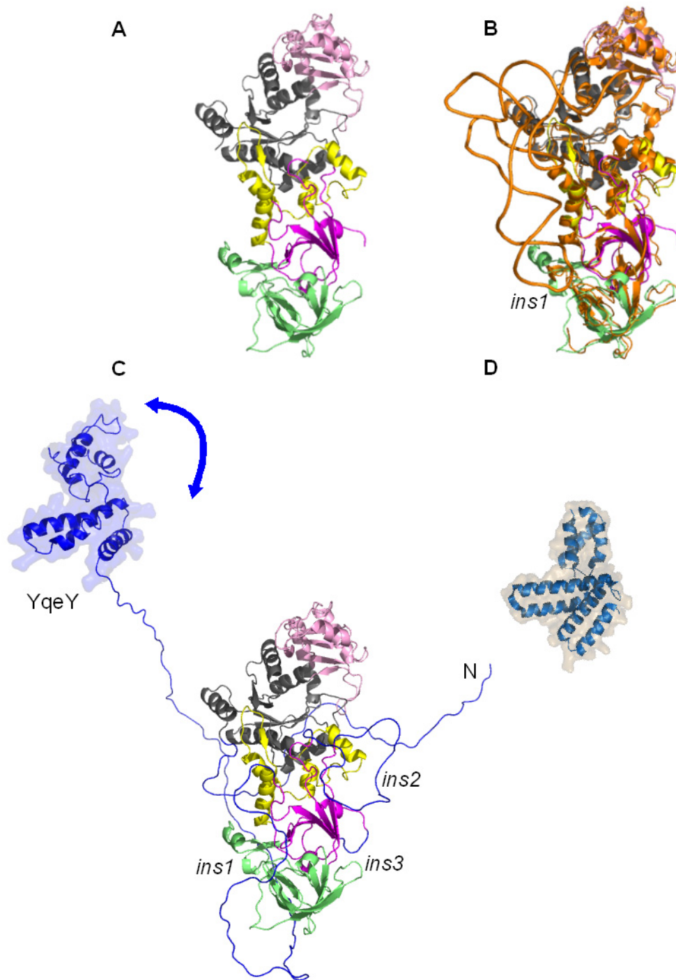
Figure II. 2 : GlnRS-Dr, une enzyme chimérique – A, B : Architecture classique du cœur conservé. A- Structure de la GlnRS de Deinococcus radiodurans résolue à 2,3 Å de résolution (PDB_id : 2HZ7), (Deniziak et al. , 2007). Le code couleur respecte la nomenclature du système E. coli . On distingue les 2 modules du site catalytique que sont le domaine de Rossmann (DNF, DiNucleotide Fold, 47-147 :252-305, en gris) et le domaine de liaison à la tige acceptrice (ABD, Acceptor-Stem Binding Domain, 143-251, en rose pâle). Le site de liaison à l'anticodon est composé de 2 sous-domaines : le domaine proximal (PBB, Proximal \beta -barrel, 380-387 :516-633, magenta) et le domaine distal (DBB, Distal \beta -barre, 388-515, vert pâle). Les modules catalytiques et de reconnaissance à l'anticodon sont reliés par un module intermédiaire (HSB – Helical subdomain, 306-379, en jaune) La plupart des insertions (sauf ins1 ) ne sont pas visibles dans la structure. B- Superposition des structures de la GlnRS de Deinococcus et E. coli (PDB_id : 1O0B). Les codes couleurs pour la GlnRS-Dr sont les mêmes qu'en A. La GlnRS-Ec est représentée en orange clair. Le RMSD global est de 1,9 Å; l'architecture classique est conservée. C- Modèle de la GlnRS-Dr dotée des régions non visibles dans la structure. Les régions correspondant au modèle sont en bleu. Les extrémités N- et C-terminale avec le domaine Yqey (surface), les insertions ins1 et ins2 sont précisées. Le modèle a été déterminé à partir des structures de la GlnRS et de Yqey de Bacillus subtilis (PDB_id : 1NG6). D- Structure de Yqey de Bacillus subtilis .
