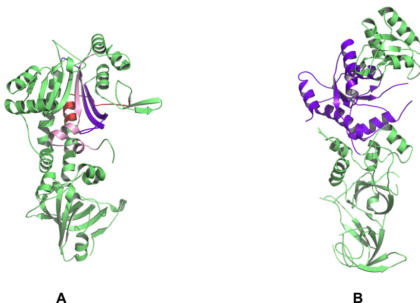
Figure 1. 2 : Mise en relief des différences d'organisation du site actif des aaRS : exemple d'une aaRS de classe II, l'AspRS de levure (A) , et de classe I, la GlnRS d' Escherichia coli (B).
