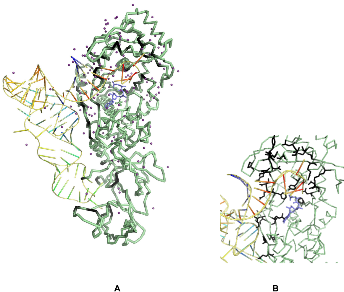
Figure I. 4 : Représentation des régions impliquées dans la discrimination de l'ARNt Gln par la GlnRS d' E. coli . Les régions impliquées pour l'ensemble de l'enzyme (A) ou uniquement dans la région du site catalytique (B) sont colorées en noir, l'enzyme en vert pâle et l'ARNt en jaune (pdb-id 1EUQ).
