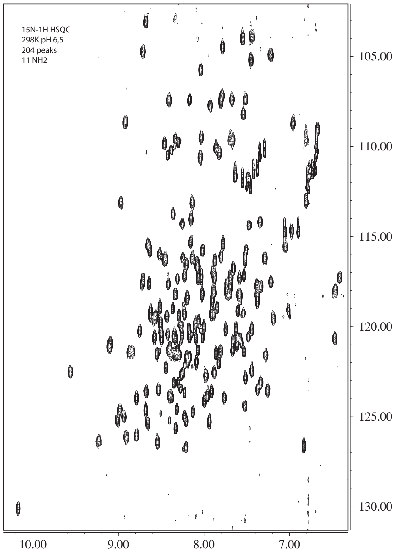
Figure II. 23 : Spectre ^1\text{H} - ^{15}\text{N} – HSQC du domaine YqeY- \Delta marqué en ^{15}\text{N} à 25°C pH 6.5. Les taches individuelles représentent les déplacements chimiques de chaque “proton amide” avec en abscisse ceux des ^1\text{H} et en ordonnée ceux des ^{15}\text{N} . On décompte 204 pics dont 11 potentiels pour les NH2 des chaînes latérales des asparagines et glutamines.
