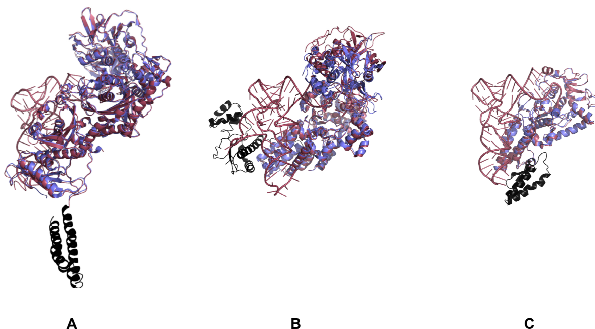
Figure I. 17 : Exemples de structures dont la résolution en présence de l'ARNt correspondant ont permis de stabiliser des domaines flexibles sous forme libre. Structures de A - la PheRS de T. thermophilus , apo ou complexée à l'ARNt Phe (1JJC et 1EIY, respectivement), B - la CysRS d' E. coli apo ou complexée à l'ARNt Cys (PDB-ID :1LI5 et 1U0B, respectivement) et C - : la LeuRS de Pyrococcus horikoshii apo ou complexée à l'ARNt Leu (1WKB et 1WZ2, respectivement). Les structures des enzymes sous forme apo et complexée sont superposées et colorées en bleu et rouge brique, respectivement. Les domaines additionnels stabilisés en présence d'ARNt sont colorés en noir.
