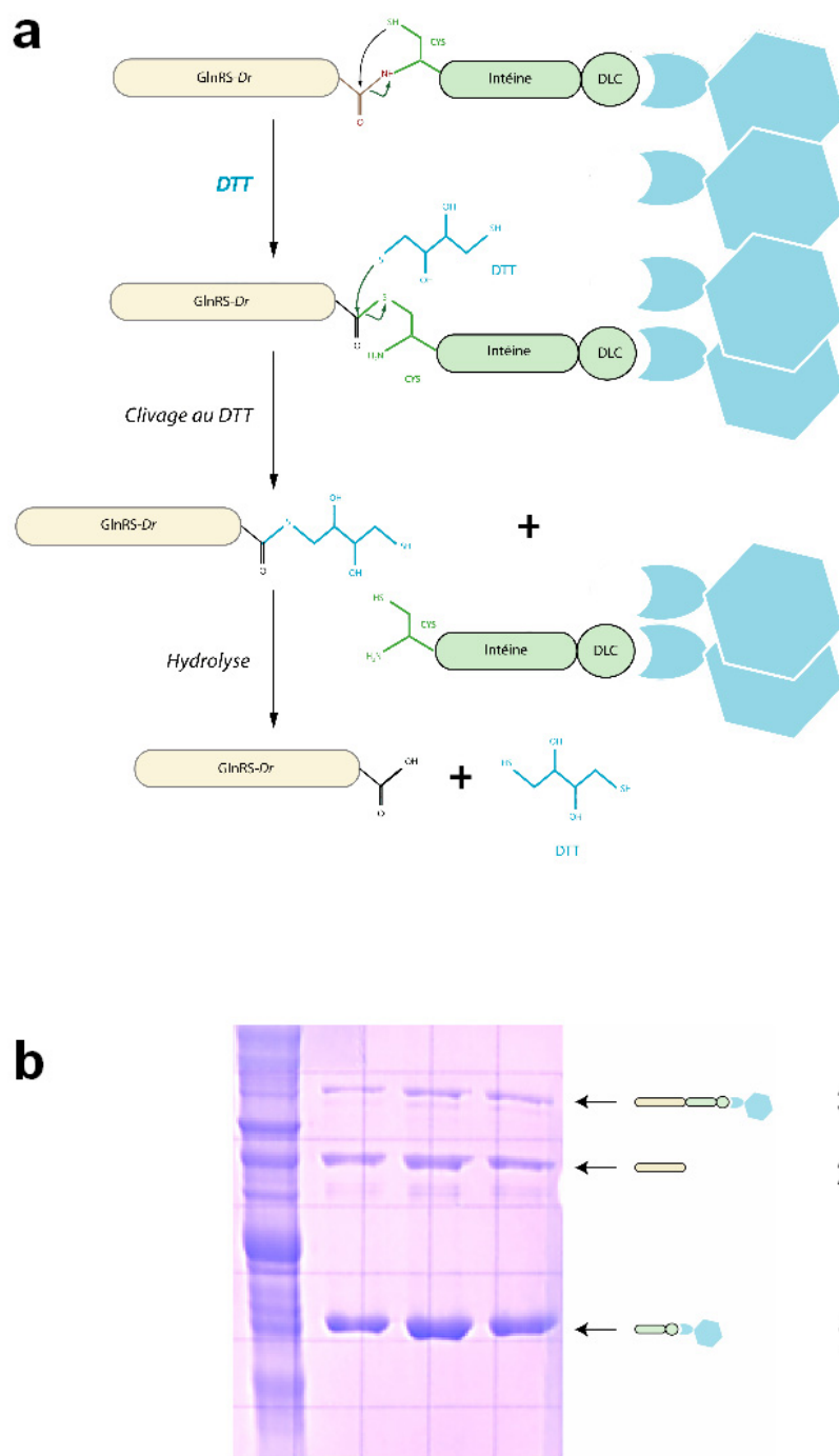
Figure III. 1 : a : Schéma de la réaction d'autoclavage entre la protéine cible (ici GlnRS-Dr) lors de l'incubation en présence de Dithio-thréitol (DTT).- b : Gel SDS en conditions dénaturante d'un extrait de matrice de chitine chargé par la construction fusionnée GlnRS-Intéine et incubée durant la nuit à 50mM DTT. Le produit de la réaction d'autoclavage est constitué de l'intéine qui reste accrochée aux billes de chitine (intéine en vert, billes en bleu, (1.) et de la protéine d'intérêt. Ici, la GlnRS est décrochée de la matrice et élue par simple lavage (GlnRS-Dr, en jaune, 2.). La réaction n'étant pas totale, il subsiste parfois sur la matrice un produit non encore clivé (annoté 3., représentant GlnRS-intéine-chitine).
