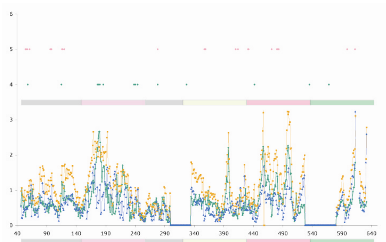
Figure II. 20 : Représentation graphique de la distance entre les résidus des structures 2 à 2.
