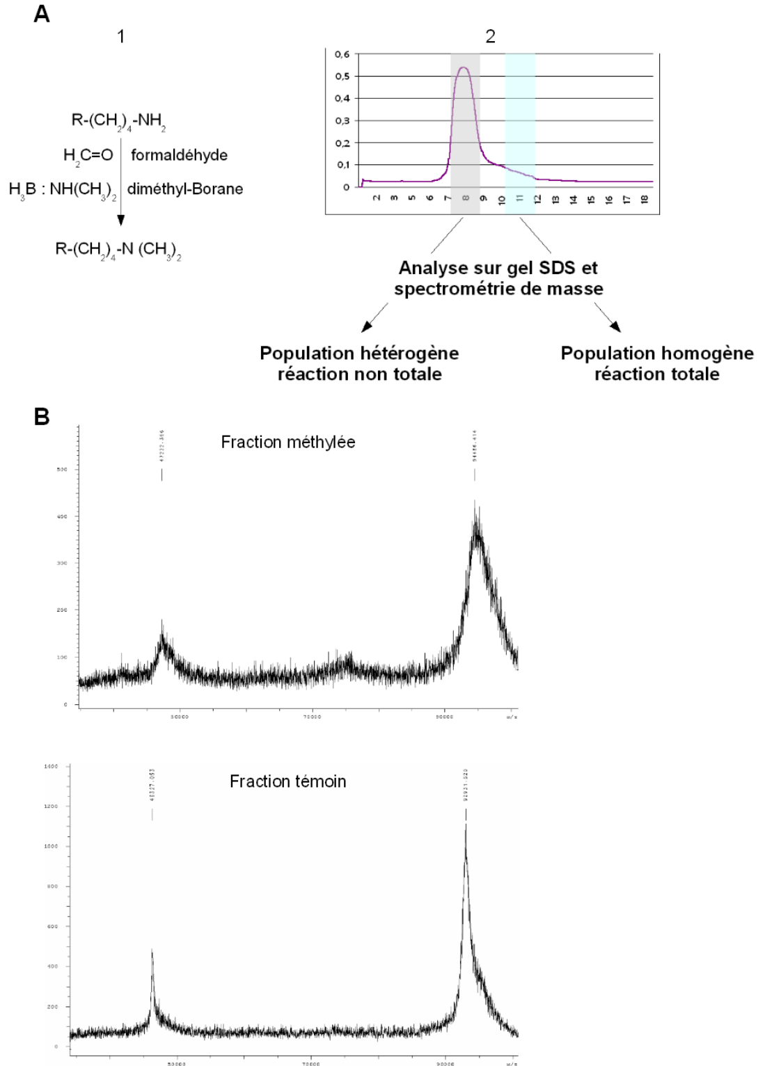
Figure II. 7: Schéma du protocole suivi pour la méthylation des lysines. A : 1 - Réaction opérée sur la chaîne latérale des Lysines ( \text{R}-(\text{CH}_2)_4-\text{NH}_2 ). En présence de formaldéhyde et de diméthyl Borane, les \text{NH}_2 terminaux sont méthylés. 2. Profil de la chromatographie d'exclusion de taille de la GlnRS traitée. Les fractions sont analysées sur gel SDS en conditions dénaturantes et en spectrométrie de masse. La population majoritaire est très hétérogène (fraction 7 à 9). Une petite part de la fraction traitée (11-12) est effectivement méthylée et peut-être séparée sur chromatographie d'exclusion de taille. B : Spectres MALDI-TOF en spectrométrie de masse de la fraction méthylée de la GlnRS (11-12, Fraction méthylée) et de la GlnRS non traitée (Fraction témoin). On observe un décalage de 1500 Da entre les deux échantillons. Les mesures sont effectuées sur un appareil Brucker Biflex III. Les morceaux de gel correspondant sont découpés et digérés à la trypsine pour les mesures (Voir aussi le chapitre Matériel et Méthodes , V. A).
