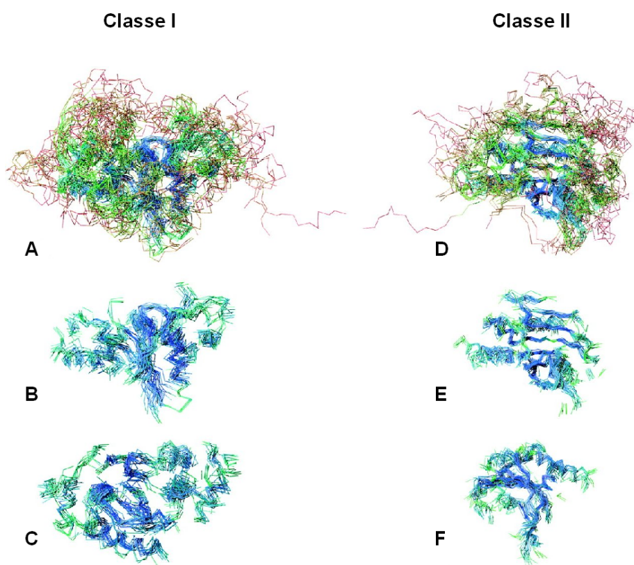
Figure I. 6 : Superposition des domaines catalytiques des classes I et II : vers la définition d'un domaine ancestral? Les structures de tous les domaines catalytiques des aaRS ont été alignées séparément pour les classe I (a à c) et II (dà f), basé sur les alignements structuraux. Les synthétases des deux classes ne sont pas liées structuralement. Le code couleur suit le degré de conservation structurale allant du brun (le moins conservé) au bleu foncé (le plus conservé). Le panneau inférieur de la figure (bc, ef) montre, dans différentes vues, le cœur conservé des domaines catalytiques sans les insertions. Schéma d'après (O'Donoghue et Luthey-Schulten, 2003).
