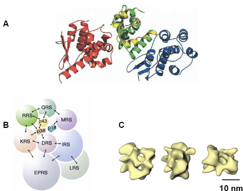
Figure I. 7 : Structures tridimensionnelles et modèles de complexes multisynthétasiques d'eucaryotes inférieurs et supérieurs. A - Modèle du complexe ternaire MetRS-N - Arc1P-N - GluRS-N de Saccharomyces cerevisiae . Le domaine d'interaction de la MetRS (MetRS-N) est représenté en bleu, de la GluRS (GluRS-N) en rouge et les domaines Arc1p correspondants (MetRS-N - Arc1P-N et Arc1P-N - GluRS-N) en vert et jaune, respectivement. Le domaine d'interaction de la protéine Arc1p exhibe des sites de liaison avec ces aaRS qui lui permettent de les lier simultanément ou indépendamment (Simos et al. , 1998). Ce domaine (GST) est souvent retrouvé chez les protéines impliquées dans le complexe multisynthétasique eucaryote. Figure d'après (Simader et al. , 2006b). B - Schéma d'interaction des éléments du complexe multisynthétasique des eucaryotes supérieurs. Le schéma utilise le code acide aminé à une lettre (Lee et al. , 2004). C - Structure tridimensionnelle du complexe obtenue par cryomicroscopie électronique (Wolfe et al. , 2003) respectivement et de gauche à droite en vue de face, vue de profil (rotation de 90° sur l'axe vertical) ou du dessus (rotation de -90° sur l'axe horizontal).
