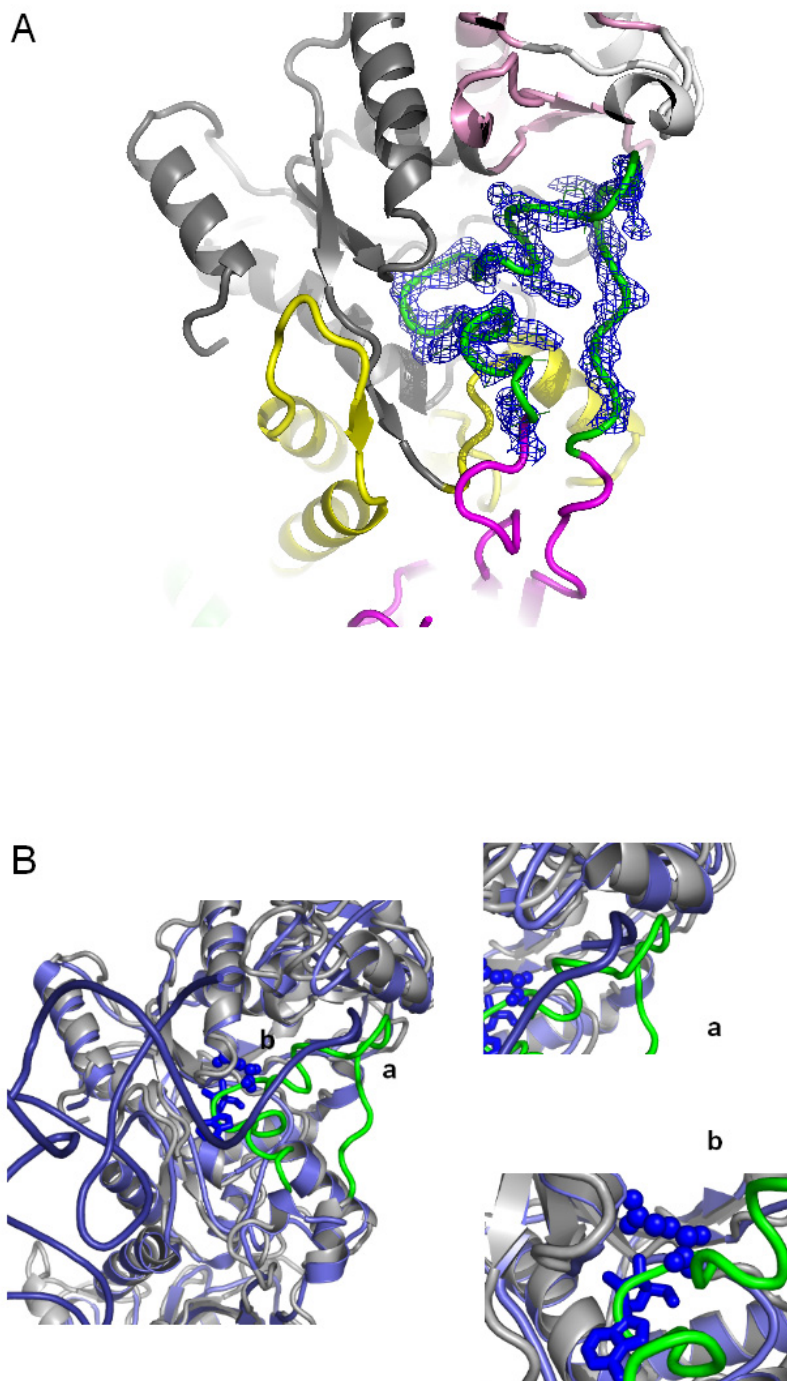
Figure II. 13 : Vue rapprochée du site actif de la GlnRS-Dr dans sa conformation fermée. Celle-ci est observée lorsque la GlnRS-Dr est co-cristallisée en présence de glutamine. Les codes couleurs des domaines de la GlnRS sont identiques à ceux de la figure II. 2 . La boucle d'insertion est représentée en vert clair dans toutes les figures. (A) Représentation de la conformation fermée du site actif de l'enzyme. La carte différence (Fo-Fc) de la densité électronique de la boucle est contourée à 2,5 \sigma et représentée en bleu; (II) superposition de la structure de la GlnRS-Dr (gris clair) avec celle d' E. coli (bleu électrique) complexée à l'ARNt Gln , la glutamine et l'AMP. (B, a) : vue rapprochée de la zone de l'extrémité 3' CCA de l'ARNt (bleu foncé) et de la boucle du site actif GlnRS-Dr (vert clair). (B, b) : vue rapprochée du site de reconnaissance de l'acide aminé et visualisation de la boucle d'insertion dans cette zone (PDB_id : 1O0B).
