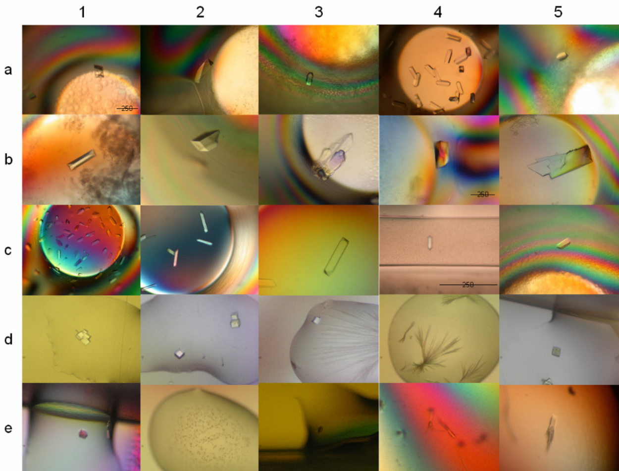
Figure II. 6 : Tableau des conditions de cristallisation et exemples des cristaux obtenus – Lignes a ; b : Exemples de cristaux de la GlnRS native (a1-c5) cristallisée en batch, avec gel d'agarose (b1-5; c2,3), en capillaires (c4), de la GlnRS-ΔC (d1-5), de YqeY-λ ou de la GlnRS en complexe avec l'ARNt Gln transcrit (e4-5). Les cristaux obtenus ont été testés à l'ESRF (European Synchrotron Radiation Facility) de Grenoble. Les co-cristaux de GlnRS et des petits ligands ont permis d'enregistrer 4 jeux complets de données entre 1,9 et 2,5 Å en présence de glutamine, et de 2 analogues d'adénylate (QSI et QOL). Les cristaux obtenus en présence de la GlnRS-ΔC ont conduits à l'enregistrement d'un jeu de données à 1,9 Å de résolution. Les cristaux obtenus en présence d'ARNt Gln ne diffractent pas au-delà de 25 Å. Les données de la GlnRS-QOL et la GlnRS-ΔC ont fait l'objet d'une analyse préliminaire.
