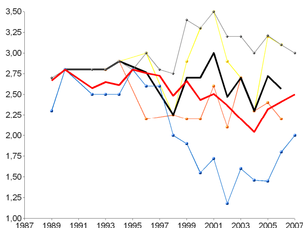
Figure I. 14 : Représentation graphique de la moyenne des résolutions des structures cristallographiques. La moyenne globale est représentée en rouge, la moyenne des structures résolues en complexe en noir. Les minima sont représentés en bleu et orange pour les résolutions globales et en complexe, respectivement, les maxima sont en jaune (global) et gris (complexe). Si la résolution moyenne globale ne diminue pas nettement, l'historique des résolutions maximales augmente sans contestes vers des valeurs de résolution atomique.
