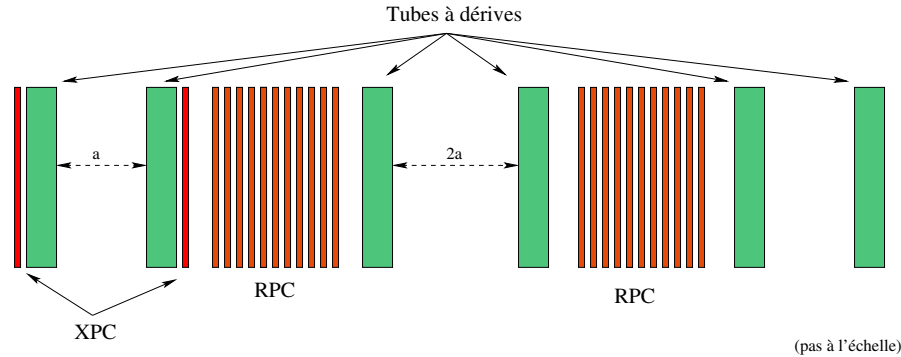
FIG. 3.18: Disposition des détecteurs de précision au sein et aux alentours du spectromètre.
