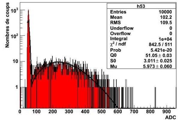
FIG. 4.34 : Exemple de distribution obtenue lors de l'étalonnage avec le spectromètre à électrons.
