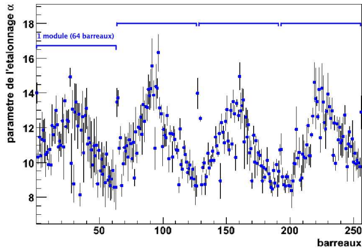
FIG. 5.60 : Paramètre de l'étalonnage \alpha en fonction du numéro de barreaux pour les 4 côtés d'un mur.
