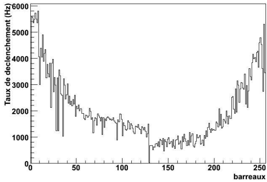
FIG. 5.49: Taux de comptage (Hz) pour les barreaux verticaux (septembre 2007).
