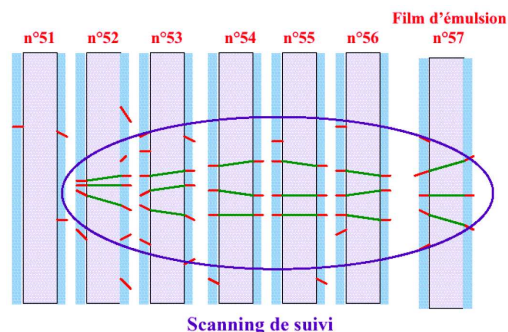
FIG. 3.22 : Scanning de suivi : il s'effectue de l'arrière à l'avant de la brique. Les traces de base sont suivies à partir de la dernière émulsion jusqu'au point d'arrêt indiquant un éventuel vertex.
