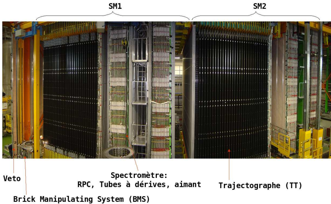
FIG. 3.9: Vue d'ensemble du détecteur OPERA dans le Hall C du LNS.
