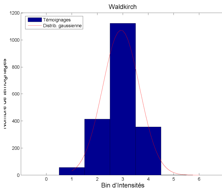
Figure 7: Répartition spatiale des SQI selon leur valeur pour le séisme de Waldkirch et histogramme du nombre de témoignage en fonction des valeurs des SQI. Les étoiles rouges représentent les épacentres des séismes. Les points bleus figurent les témoignages individuels collectés pour les trois séismes. Les triangles rouges représentent les stations accélérométriques du RAP qui ont enregistré les séismes et les cercles rouges sont des zones de 10km de rayon autour des stations.
