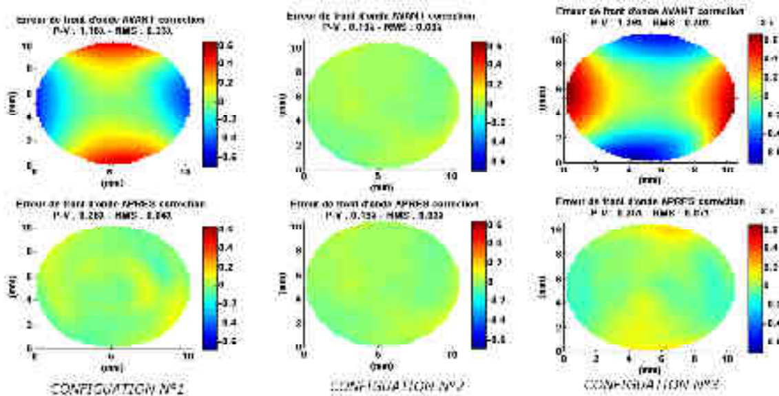
Figure D.16 : Erreur de front d'onde obtenue par la mesure des fronts d'onde restitués avant et après application de la correction adaptée pré-calculée. Une centaine d'acquisitions est prise en compte.
