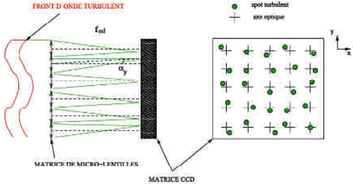
Figure A.11 : Principe de fonctionnement d'un analyseur de front d'onde de type Shack-Hartmann [86]
