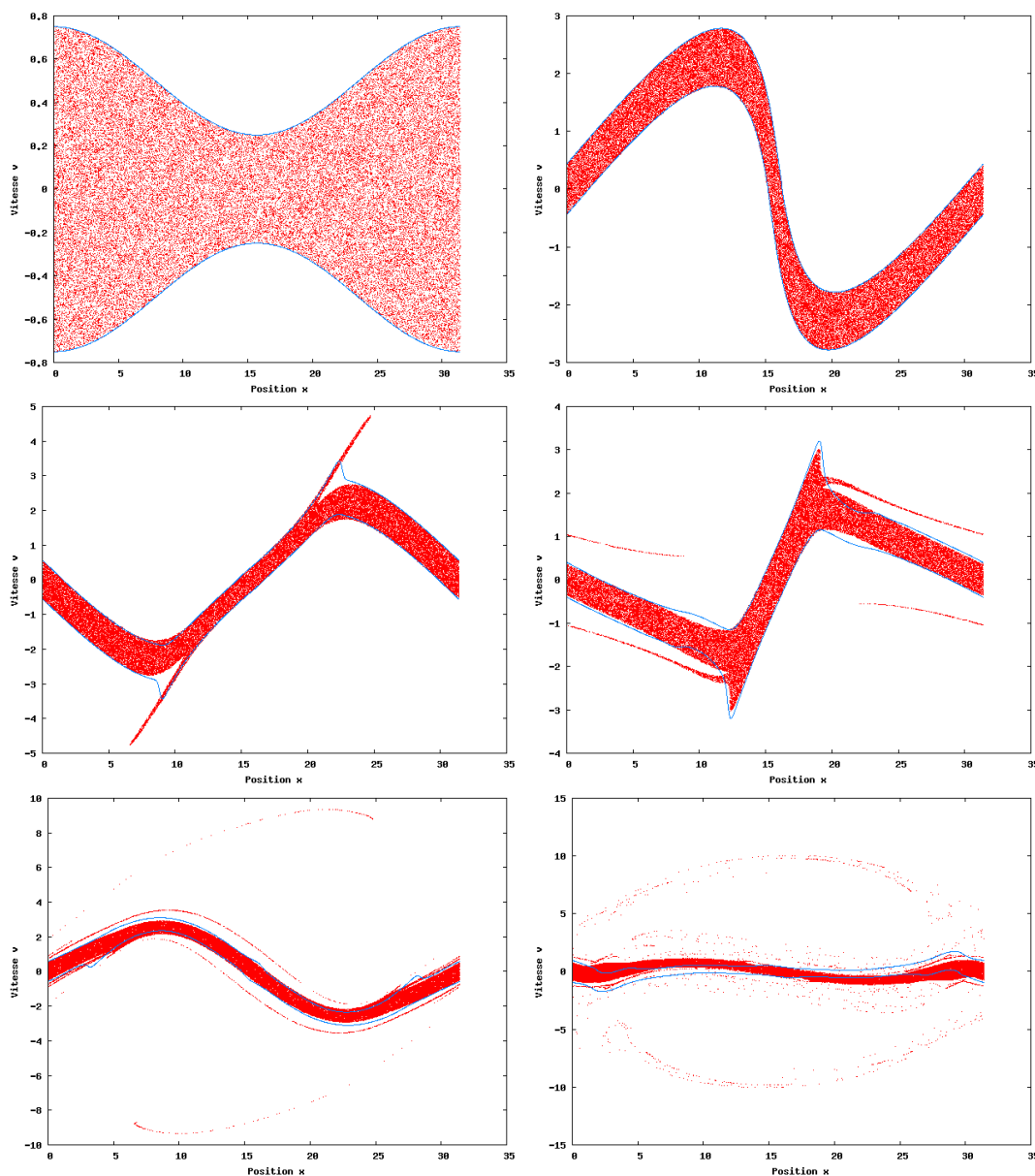
FIGURE 3.14 – Solution décrite par un water-bag - v_1^\pm (en bleu) et particules (en rouge) : t = 0, 2, 5, 10, 20 et 50 (de gauche à droite et de haut en bas).
