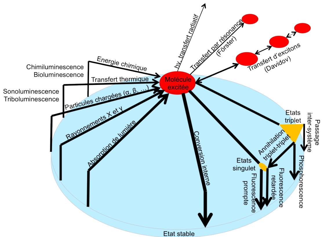
FIGURE 2.8 – Différents mécanismes d'excitation et désexcitation d'une molécule.
