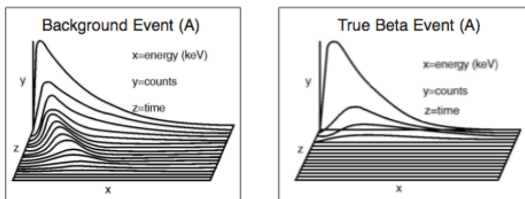
FIGURE 4.4 – TR-PDA [Passo 2002] ( Time resolved pulse decay analysis ). Méthode alliant une analyse temporelle à la discrimination, ce qui permet de différencier les évènements du fond des vrais évènements \beta .
