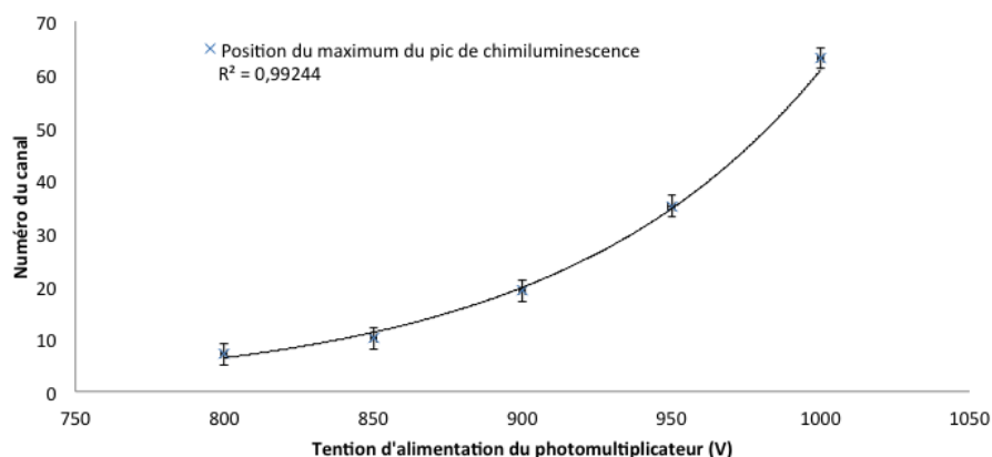
FIGURE 2.15 – Variation de la position du pic de chimiluminescence (Fig. 2.14) en fonction de la tension avec un ajustement en loi puissance, avec un coefficient de détermination R^2 à 99,244%.
