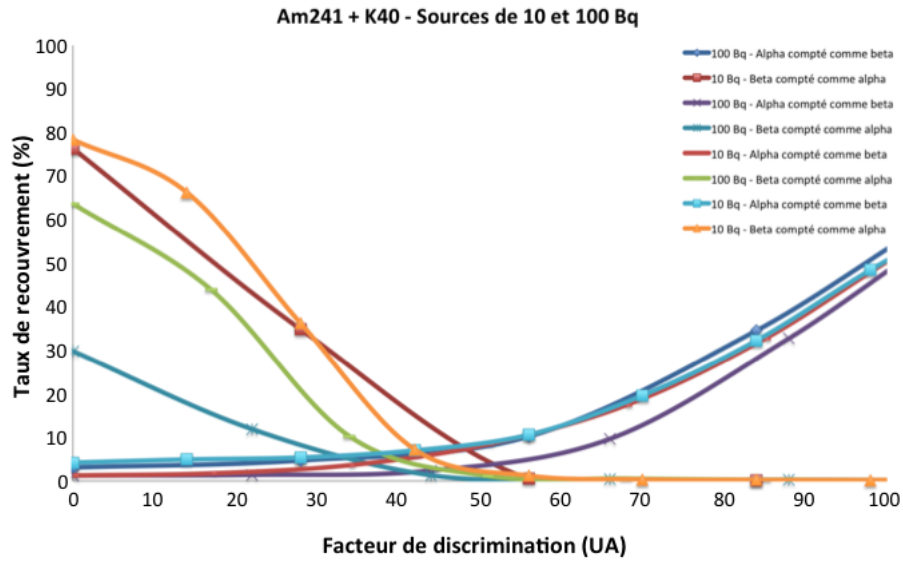
FIGURE 4.7 – Taux d’interférence pour deux sources ^{241}\text{Am} + ^{40}\text{K} de 10 et 100 Bq.
