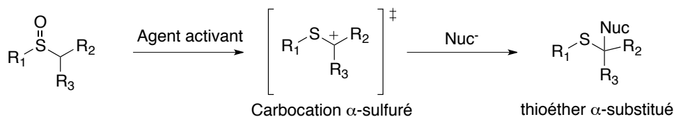
Schéma 91 : Réaction générale du réarrangement de Pummerer
