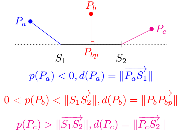
FIGURE 6.7 – Calcul de distance d'un point à un segment [S_1S_2] en fonction de la position du projeté de ce point sur l'axe du segment. Le projeté du point P_a (resp. P_c ) est à l'extérieur du segment. La distance de P_a (resp. P_c ) au segment est égale à sa distance euclidienne au point S_1 (resp. S_2 ). Le projeté P_{bp} du point P_b est à l'intérieur du segment. La distance de P_b au segment est égale à sa distance euclidienne au point P_{bp} .
