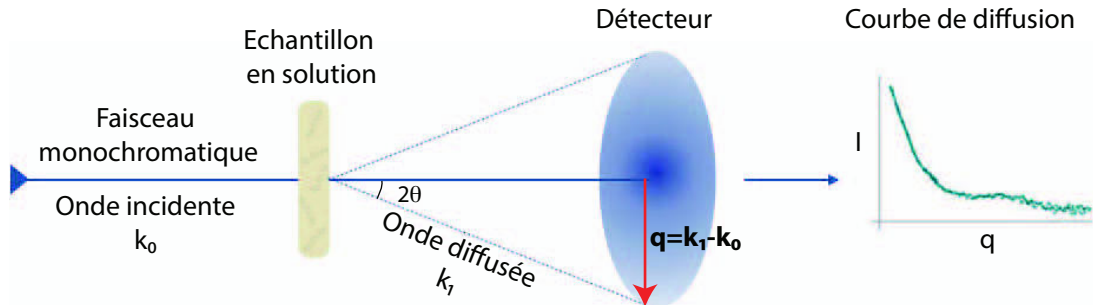
Figure 4.10 – Mesure de diffusion des rayons X aux petits angles (SAXS).
