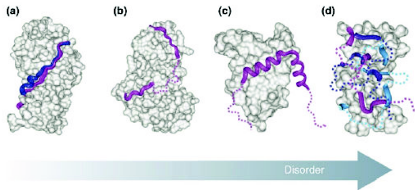
Figure 4.7 – Différents types de complexes impliqués dans les interactions protéine-protéine mettant en jeu des IDPs. L'IDP est représentée en couleur alors que la surface du partenaire est représentée en gris. (a) exemple d'un complexe polymorphique où plusieurs conformations sont présentes dans l'état lié avec le même partenaire. (b) modèle clamp : un segment désordonné sert de linker entre deux motifs d'interaction ordonnés et maintient leur liberté conformationnelle dans l'état lié de l'IDP. (c) modèle flanquant : une région adjacente à un motif d'interaction contribue à la stabilité du complexe en établissant des contacts transitoires, et (d) modèle random : la protéine reste désordonnée sur toute sa longueur pendant l'interaction. Le désordre devient de plus en plus prééminent en allant de (a) vers (d). Figure extraite de [Tomba 2008].
