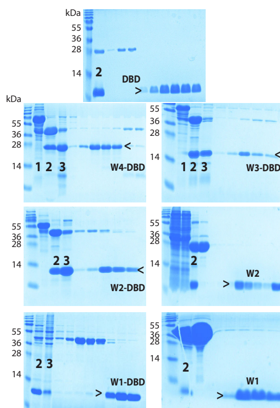
Figure 6.9 – Etapes de purification des différents polypeptides en fusion avec l'étiquette MBP. La piste 1 correspond à la protéine recombinante ; 2 correspond au clivage par l'enzyme TEV et 3 à l'étape d'ultracentrifugation. Les noms des différents polypeptides sont indiqués sur les gels SDS-PAGE au niveau des pistes correspondantes à l'étape de gel filtration.
