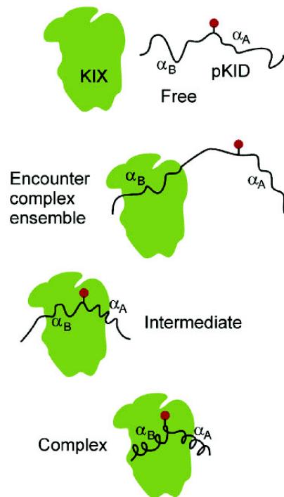
Figure 4.6 – Schéma du repliement induit du domaine phosphorylé KID (pKID) du facteur de transcription CREB lors de l'interaction avec le domaine KIX du coactivateur de la transcription CBP/p300. pKID est désordonné en solution et interagit avec KIX via son extrémité C-terminale pour former un complexe intermédiaire dynamique. S'en suit la liaison sur toute sa longueur et son repliement en deux hélices- . Figure extraite de [Wright 2009].
