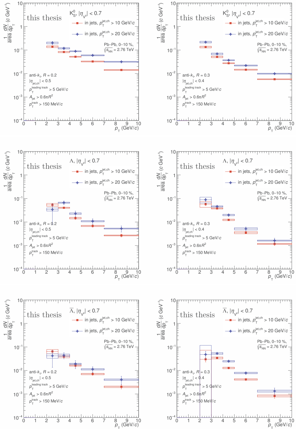
FIGURE 1 – Les spectres des particules V^0 dans les jets chargés dans les collisions Pb-Pb centrales (0-10%) à \sqrt{s_{NN}} = 2.76 \text{ TeV} enregistrées en 2011, comparés pour R = 0.2 et R = 0.3 .
