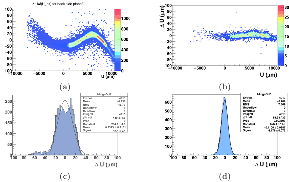
Figure 1.21 – Résultat de l'analyse de l'échelle inclinée à 36^\circ : 1.21a résidu point d'impact/trace selon la direction u en fonction de la position du point d'impact dans la même direction avant la correction, 1.21b résidu selon u en fonction du point d'impact dans la même direction après prise en compte de la déformation, 1.21c distribution des résidus point d'impact/trace avant correction et 1.21d distribution des résidus après correction.
