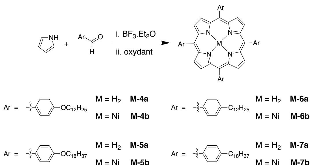
Schéma 1. Synthèse des porphyrines M-4 , M-5 , M-6 et M-7
