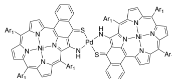
M = Ni M-7b
