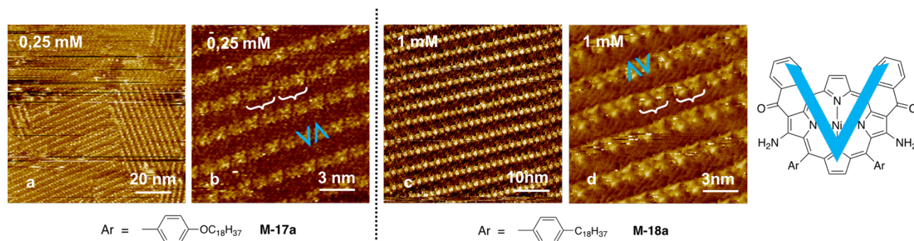
Figure 13. Images STM des assemblages de M-17a et M-18a à l'interface HOPG-phényloctane, a) I = 1,0 pA et V = -900 mV, b) I = 1,0 pA et V = -622 mV, c) I = 1,1 pA et V = -103 mV, d) I = 1,2 pA et V = -164 mV
