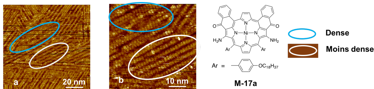
Figure 24. Images STM des assemblages des oligomères de M-17a après ajout de \text{Ni(II)} à l'interface HOPG-phényloctane, conditions STM : I = 1,2 \text{ pA} et V = -900 \text{ mV}
