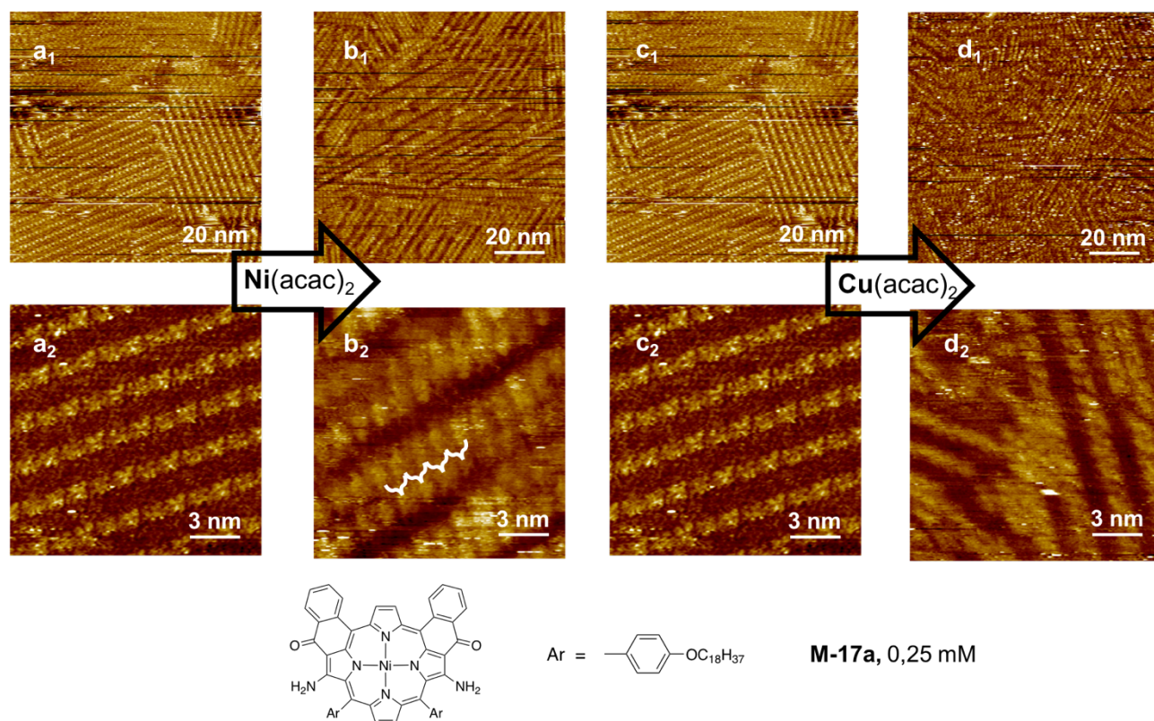
Figure 23. Images STM des assemblages des oligomères de M-17a après ajout de \text{Ni(II)} ( b_1 et b_2 ) ou \text{Cu(II)} ( d_1 et d_2 ) à l'interface HOPG-phényloctane, b_1 ) I = 1,2 \text{ pA} et V = -900 \text{ mV} , b_2 ) I = 1,2 \text{ pA} et V = -900 \text{ mV} , d_1 ) I = 1,0 \text{ pA} et V = -622 \text{ mV} , d_2 ) I = 1,2 \text{ pA} et V = -890 \text{ mV}
