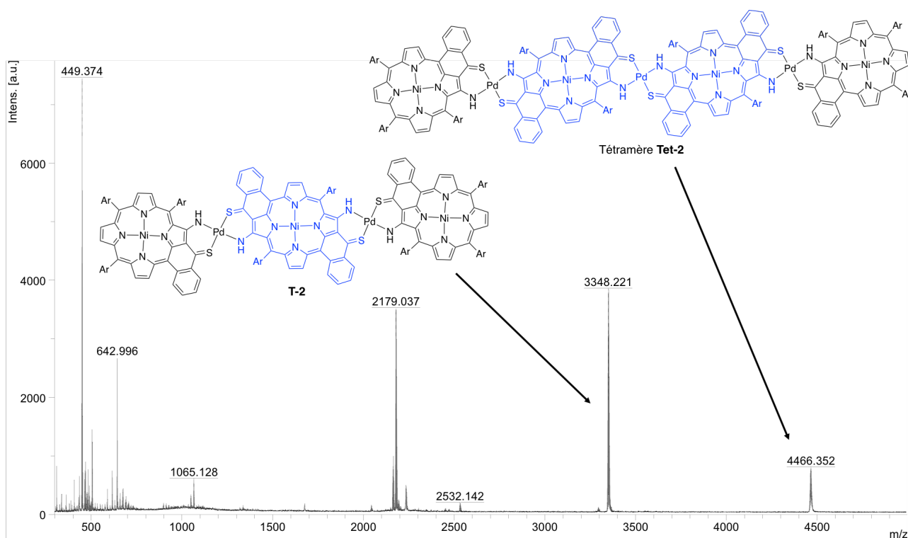
Figure 23. Spectre de masse MALDI (dithranol) après consommation des produits de départ pour la synthèse du tétramère Tet-2
