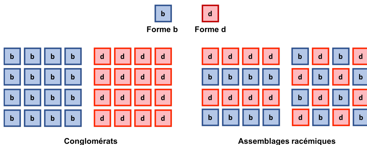
Figure 11. Assemblages racémiques 2D et conglomerats.
