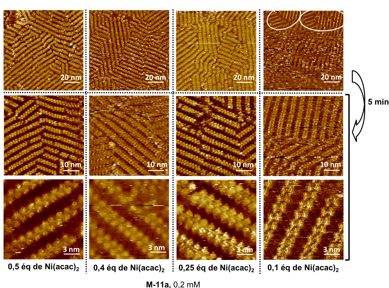
Figure 26. Variation du ratio \text{Ni}(\text{acac})_2 et M-11a pour la formation du dimère (0,05 mM)
