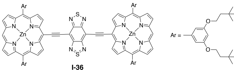
Figure 14. Porphyrines reliées par deux éthyne et un aromatique [36]
