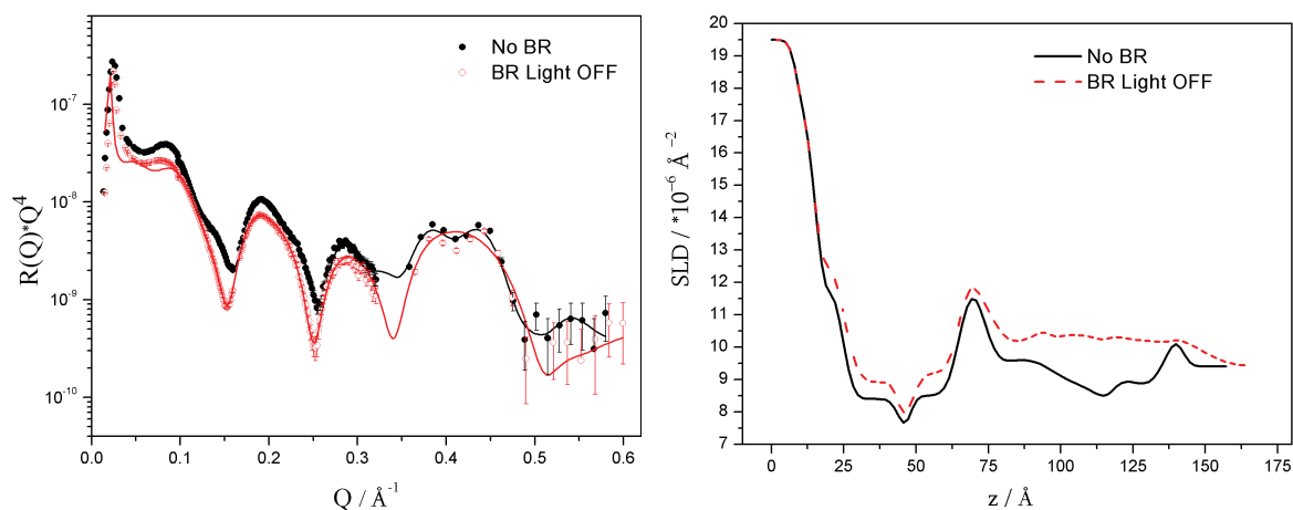
Figure VI.11 – (a) Courbes de réflectivité spéculaire de rayons X (synchrotron SOLEIL) pour une double bicouche de DSPC à 25°C avant et après l’incorporation de la BR. (b) Profils SLD correspondant aux meilleurs ajustements.
