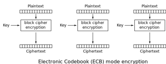
FIGURE A.1 – Chiffrement ECB, extrait de Wikipédia.
