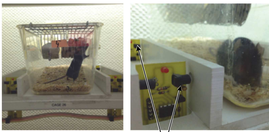
Cellules photoélectriques
