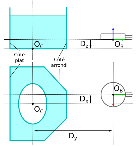
FIGURE 3.5 – Position de la base du robot par rapport à la cuve.
