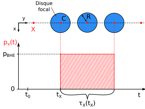
FIGURE 4.6 – Insonification statique d'un point X.
