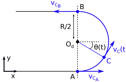
FIGURE A.20 – Paramétrage linéaire et angulaire de la trajectoire de demi-tour, entre le point A et le point B.
