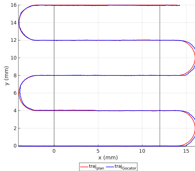
FIGURE 4.39 – Comparaison de la trajectoire théorique planifiée (en bleu) avec la trajectoire mesurée par le capteur Gocator, obtenue grâce à la détection automatique de cercle (en rouge).
