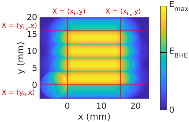
FIGURE 4.29 – Cartographie identique à celle de la Figure 4.27, avec prise en compte de la phase d'accélération ( T_{acc} = 5 s).
