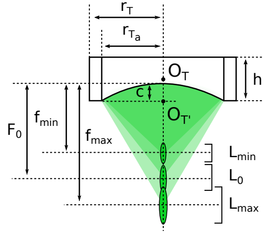
FIGURE 2.2 – Définition des paramètres du transducteur.
