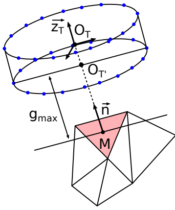
FIGURE 2.13 – La pose du transducteur, définie en partie par le point O_T , est déterminée pour une facette au barycentre M et à la normale \vec{n} . 32 points d'encombrement sont affichés pour chaque nouvelle pose testée.
