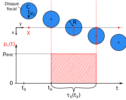
FIGURE 4.7 – Insonification dynamique d'un point X.
