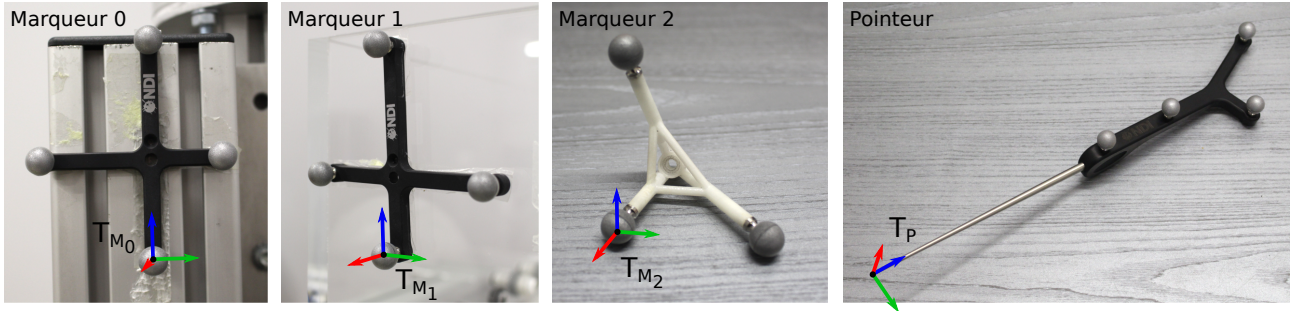
FIGURE 3.36 – Présentation des différents marqueurs utilisés pour les mesures de recalage.
