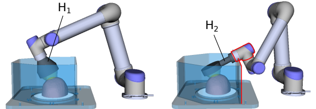
FIGURE 3.26 – Cas de collision évitée avec H_1 .
