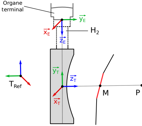
FIGURE A.6 – Définition du repère associé au transducteur pour le porte-sonde H_2 .
